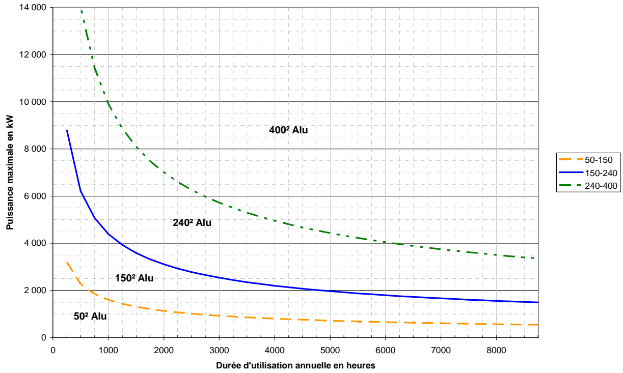
Figure 9 : Abaqués des sections économiques de câble (ne prenant pas en compte les intensités admissibles)
