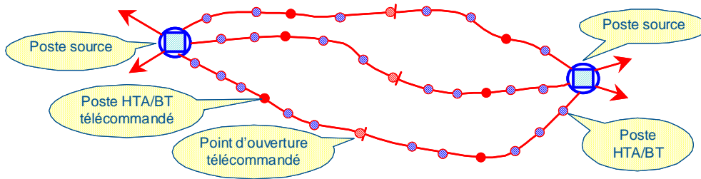
Figure 5 : exemple de structure en coupe d'artère
